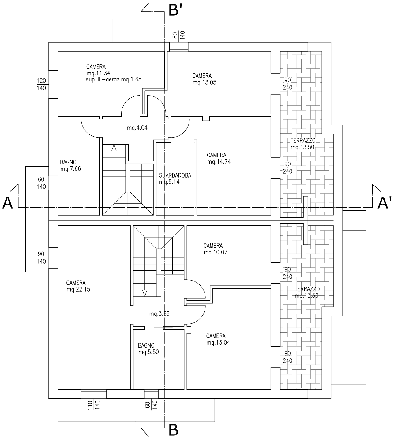
PIANTA PIANO PRIMO scala 1:100
